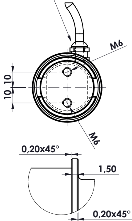
DETTAGLIO A SCALA 2 : 1
